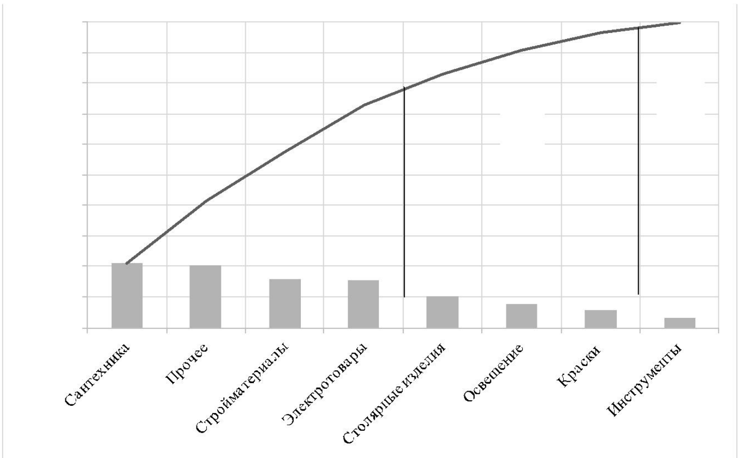
Рисунок 17. Диаграмма Парето
